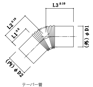
テーパ管
