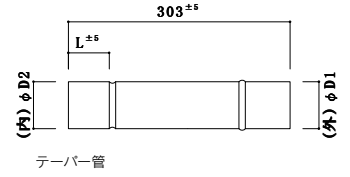
テーパ管
