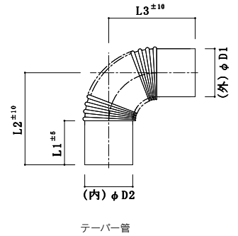
テーパ管
