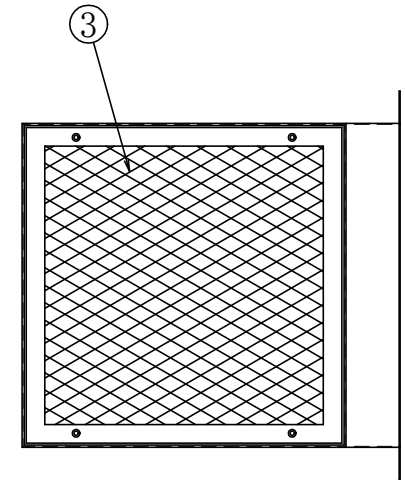
B矢視図
